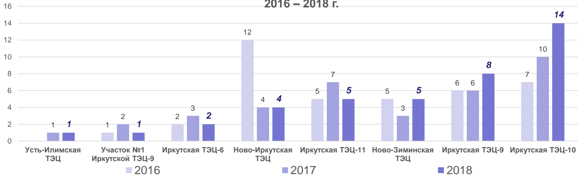
Распределение аварий за 7 месяцев по филиалам 2016 – 2018 г.
