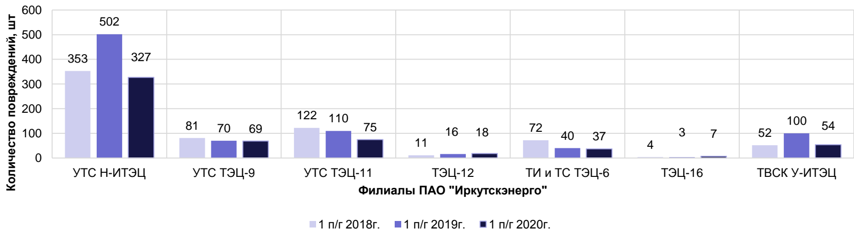
Распределение количества повреждений тепловых сетей ПАО "Иркутскэнерго" по филиалам за 2018-2020 г.г.
