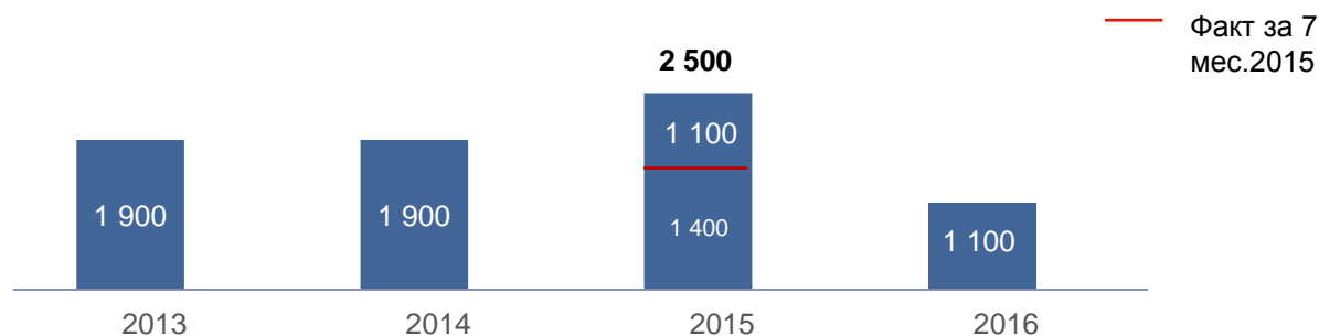
Выполнение ремонтов турбоагрегатов в 2016 году (календарный план), МВт
