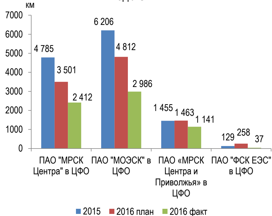
Ввод ЛЭП
