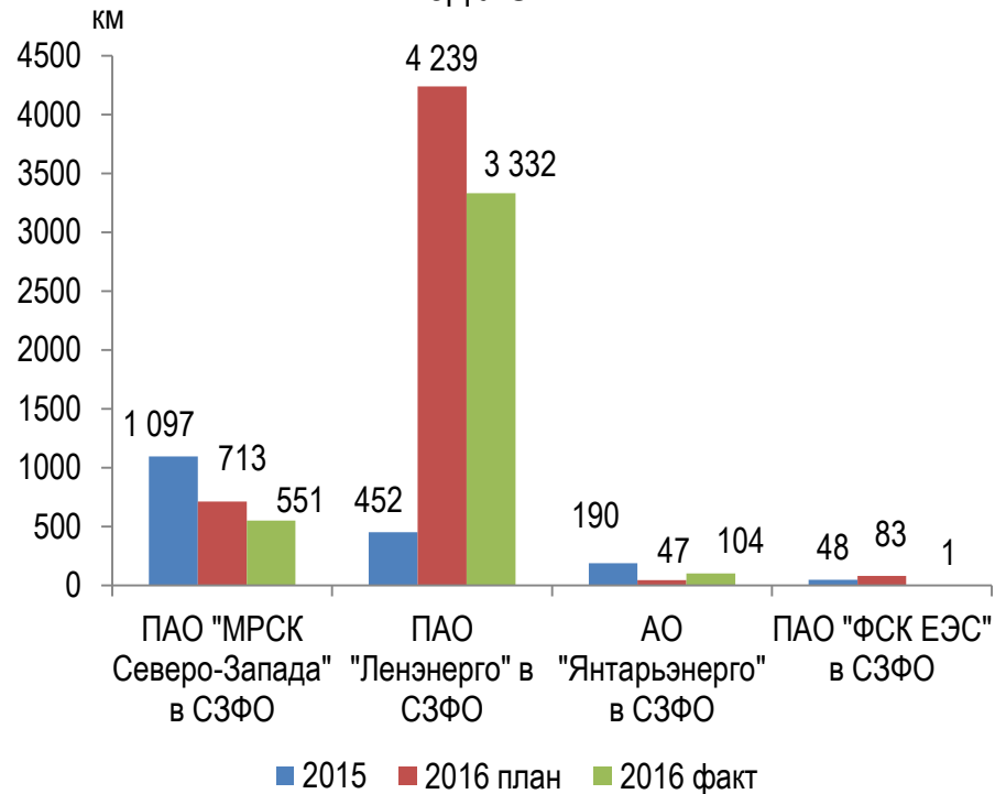
Ввод ЛЭП
