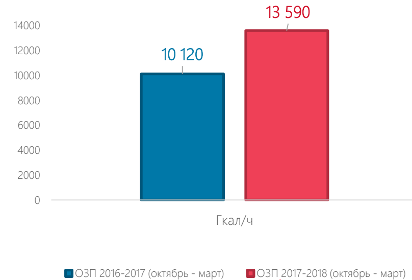
Пиковые нагрузки по отпуску тепла
