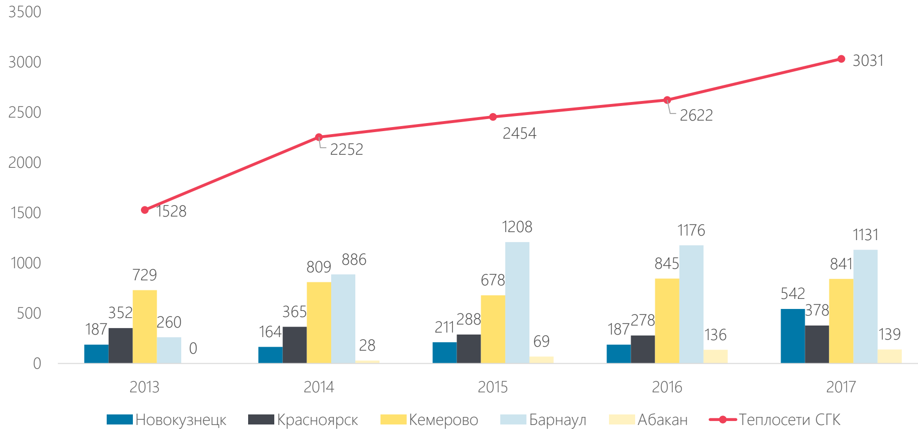
Динамика повреждаемости тепловых сетей за последние 5 лет
